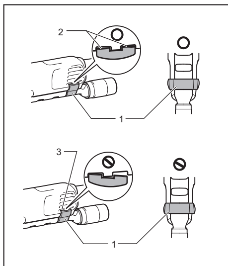
► 1. Abrazadera de boquilla 2. Protuberancias 3. Orificio
